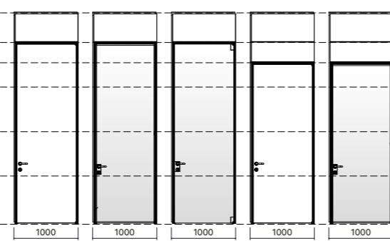
RH/LH HINGED DOORS PORTE BATTENTI DX/SX
